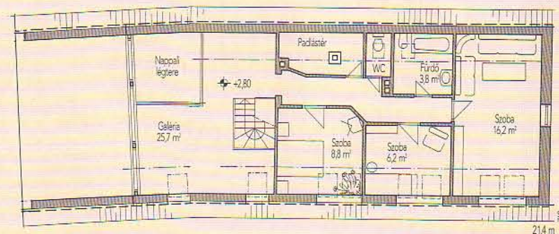
Tetőtéri alaprajz
