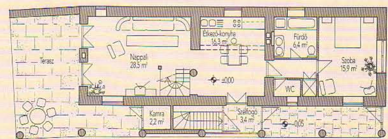
Földszinti alaprajz
